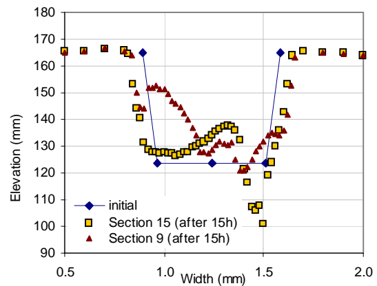
Figura 3.- Sección transversal final, ensayo 2
