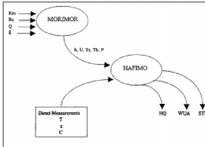
Figura 1. – Esquema de la interconexión MORIMOR-HAFIMO
