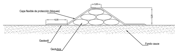
Figura 6.- Espigón proyectado
