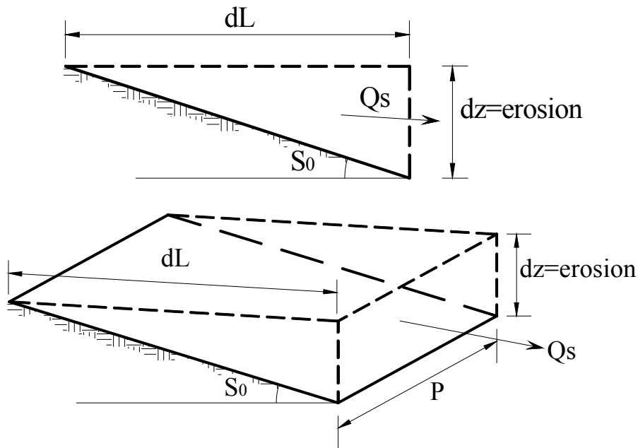
Figura 2.- Definición esquemática de hipótesis
