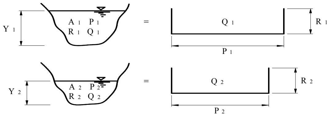
Figura 1.- Hipótesis de Manning
